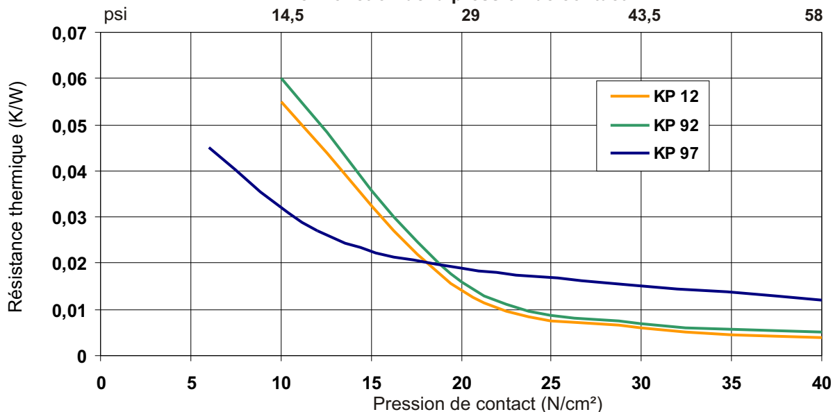
Comparaison des résistances thermiques des différentes pâtes en fonction de la pression de contact
